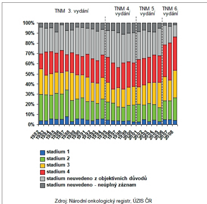
Obr. 16b – Vývoj zastoupení stadií v letech 1982–2008
