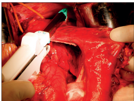
Obr. 19e – Vytváření žaludečního tubusu
